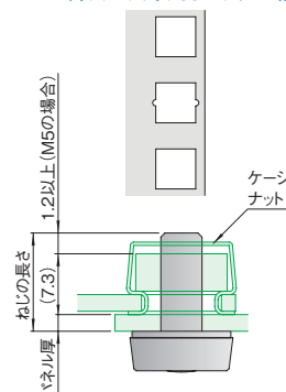
板金(四角穴) ネットワークラックSSR2シリーズ他
