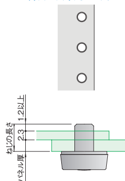
板金(M5タップ) ネットワークラックSNR2シリーズ他
