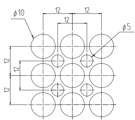
パンチング部詳細 (1 : 1) 開口率 約68%
