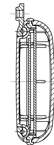
BODY-CASE ohne Vertiefung, Befestigungsöse BODY-CASE without recess, fastenings
