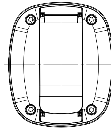
BODY-CASE ohne Vertiefung, Ansteck-Clip BODY-CASE without recess, pocket clip
