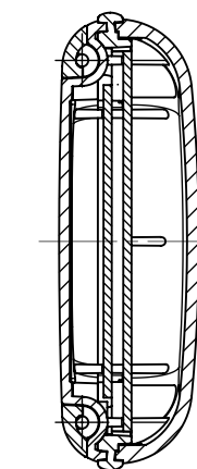
BODY-CASE ohne Vertiefung, Abdeckung und Armband BODY-CASE without recess, cover and wrist strap
