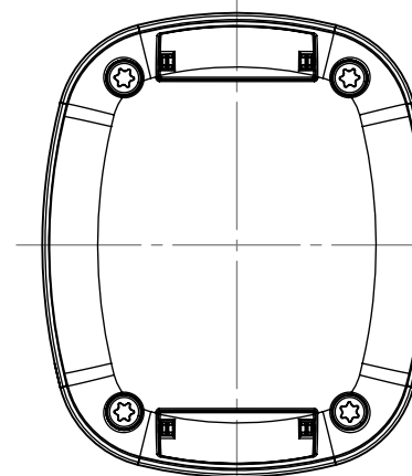
BODY-CASE ohne Vertiefung, Abdeckung und Armband BODY-CASE without recess, cover and wrist strap
