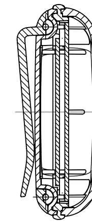
BODY-CASE ohne Vertiefung, Ansteck-Clip BODY-CASE without recess, pocket clip
