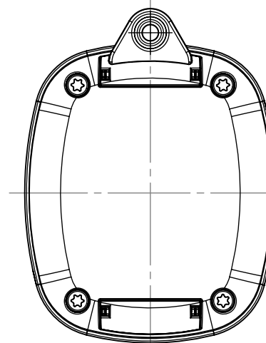
BODY-CASE ohne Vertiefung, Befestigungsöse BODY-CASE without recess, fastenings
