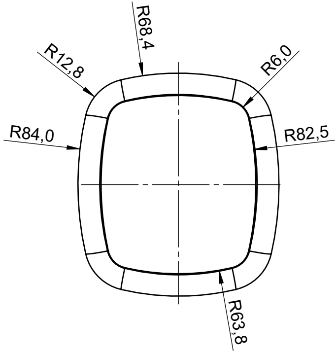
Oberteil mit Vertiefung Top part with recess
