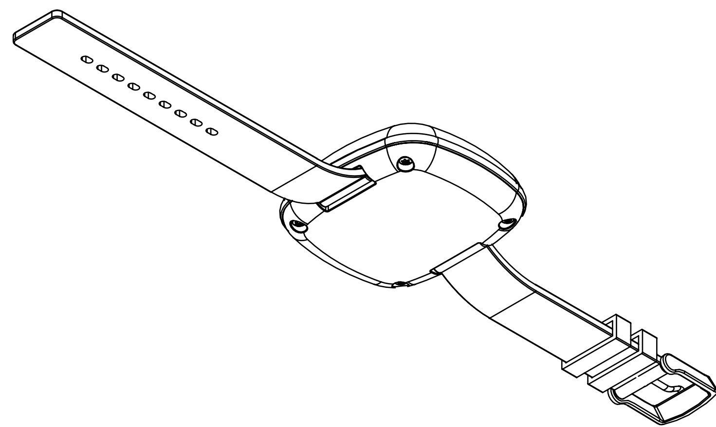
BODY-CASE mit Vertiefung und mit Armband BODY-CASE with recess and with silicone wrist strap
