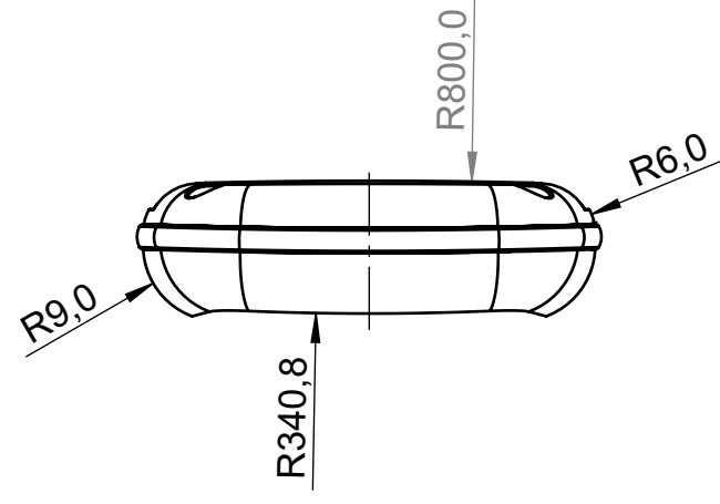
Oberteil mit Vertiefung Top part with recess
