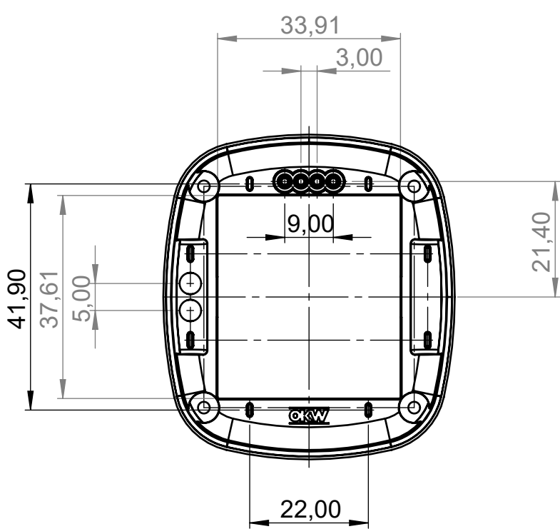
Unterteil Base part
