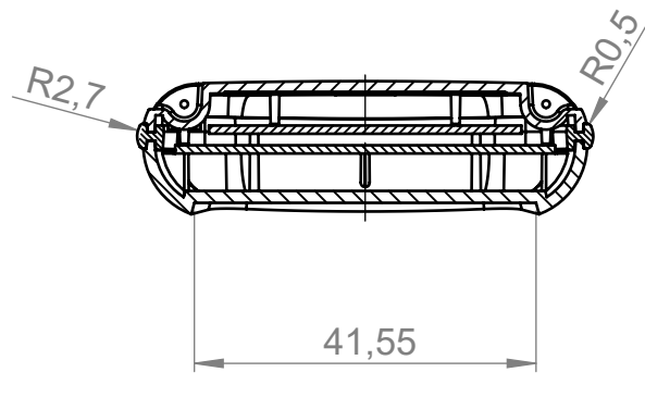
Schnitt B-B
