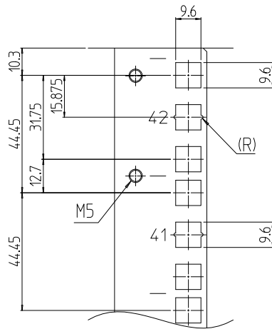
B部詳細 (1 : 2)
