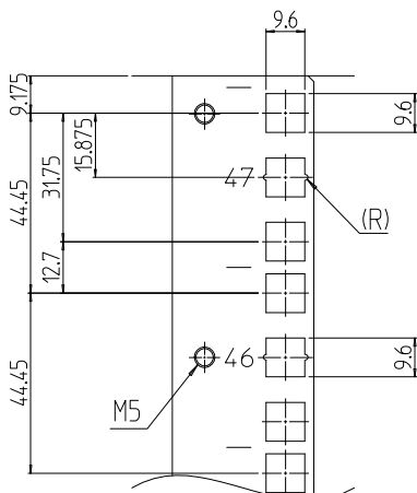
B部詳細 (1 : 2)
