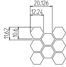
パンチング部詳細 (1 : 2) 開口率 約83% (前後ドア)
