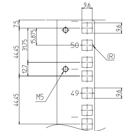
B部詳細 (1 : 2)
