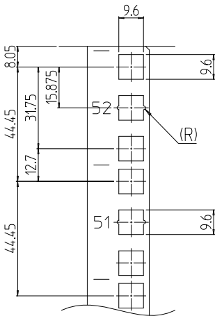
B部詳細 (1 : 2)
