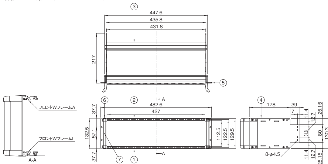
6Uダブルハイット挿抜ハンドル対応型 (FRS-2617-84IHG)
