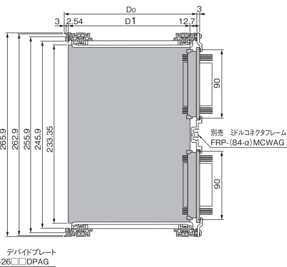
鉛直断面(正面向かって右側)
