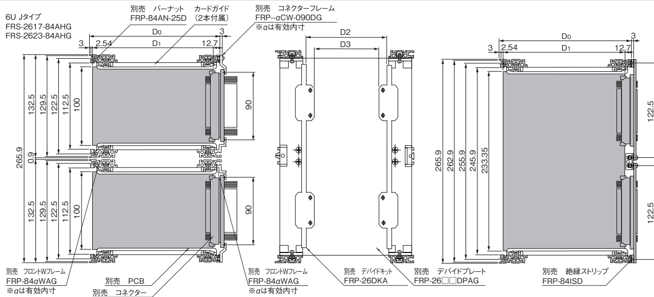
鉛直断面 (正面方向から左側)
