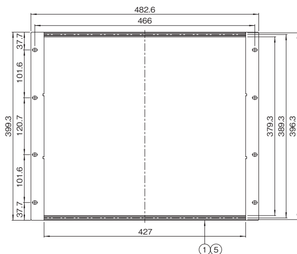
9Uトリプルハイト (FRS-39□□-84ANG/BNG)
