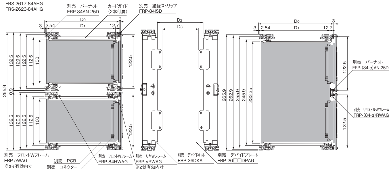
鉛直断面 (正面から左側)
