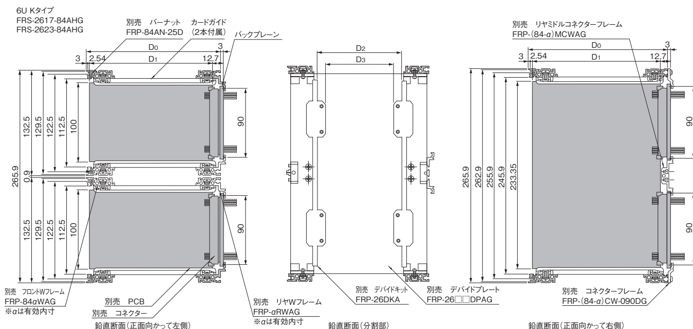
鉛直断面 (正面方向から左側)
