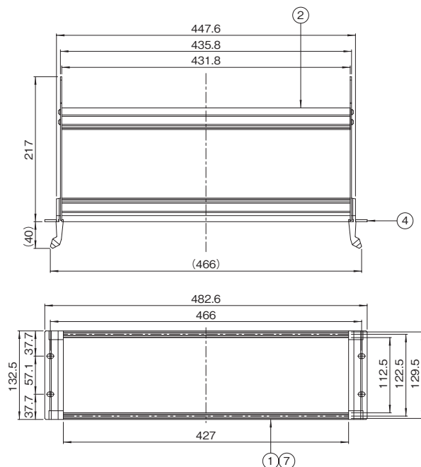
3Uシングルハイト (FRS-13□□-84AHG/BHG)
