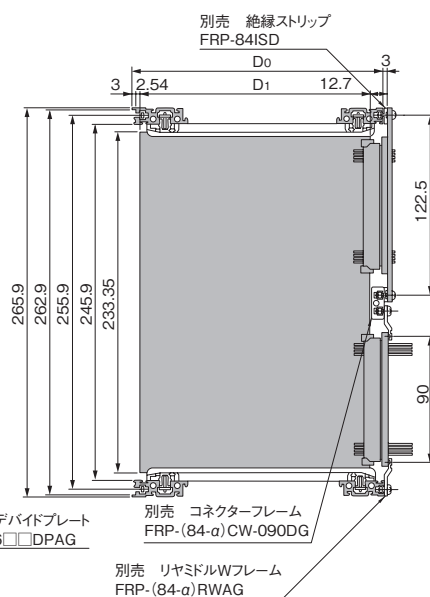
鉛直断面(正面向かって右側)
