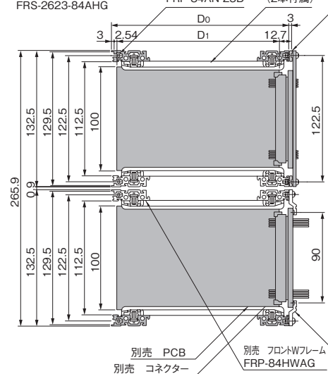
鉛直断面(正面向かって左側)
