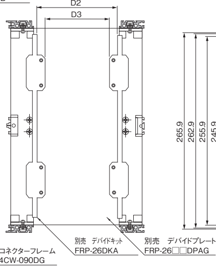
鉛直断面(分割部)
