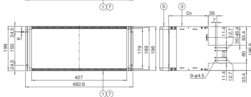
4Jハイット(FRS-20□□-84AHG/BHG)
