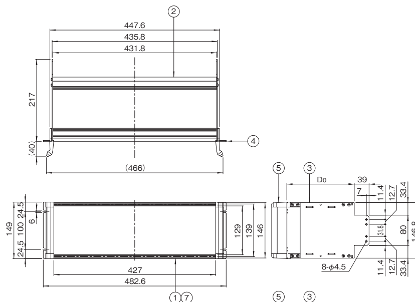
3Jハイット(FRS-15□□-84AHG/BHG)
