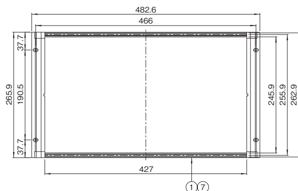
6Uダブルハイト (FRS-26□□-84AHG/BHG)
