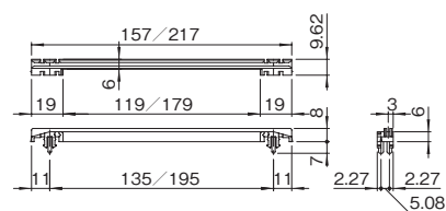
カードガイド (全機種共通)
